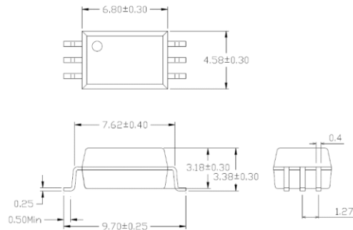
P-1.27 Type
