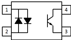
AC Input Type
